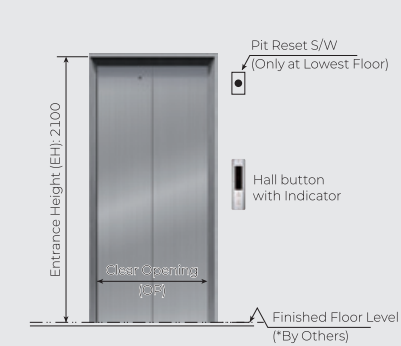
E100 TYPE (OPTIONAL)
