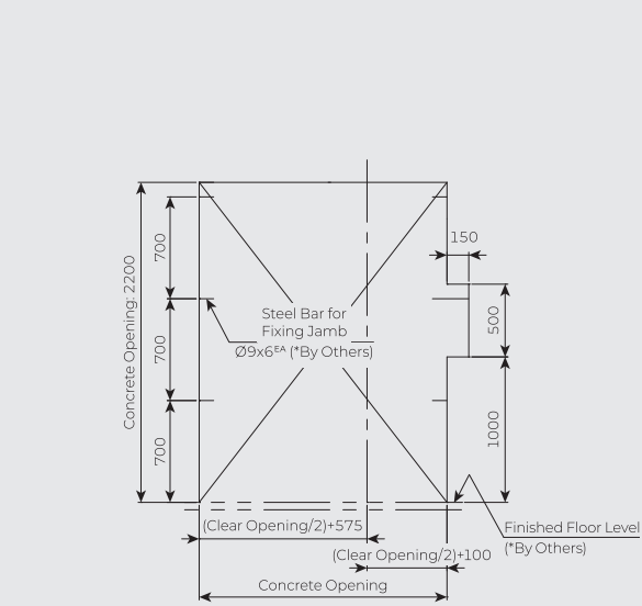
WE050 TYPE (STANDARD)
