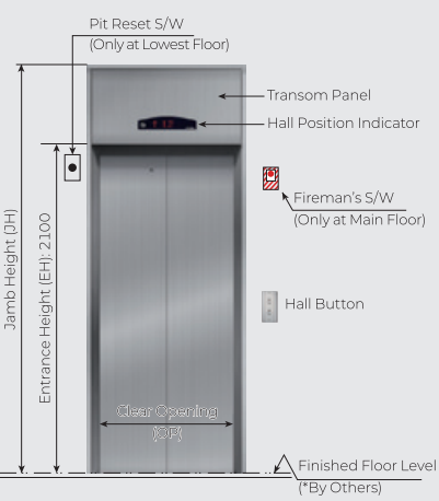
E200 TYPE (OPTIONAL)
